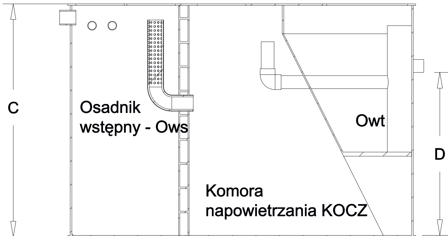
PRZEKRÓJ
